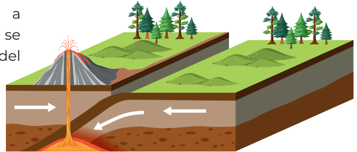
Imagen 5. Geología, San Martín Texmelucan, Puebla
